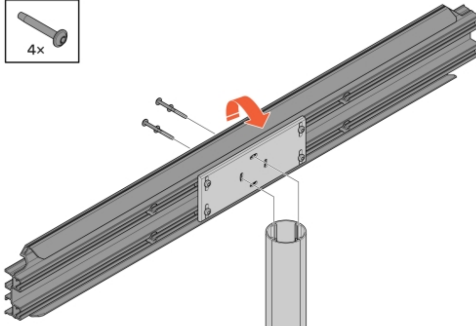
Illustration 18: Montage d'un support
