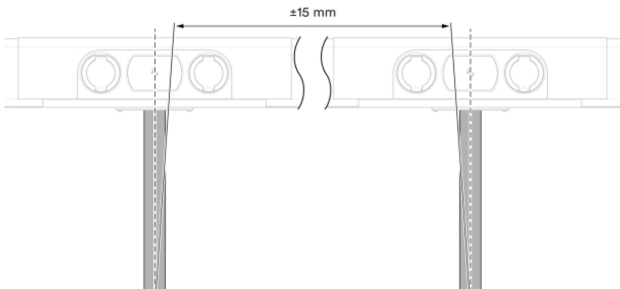
Illustration 16: Inclinaison maximale – totale
