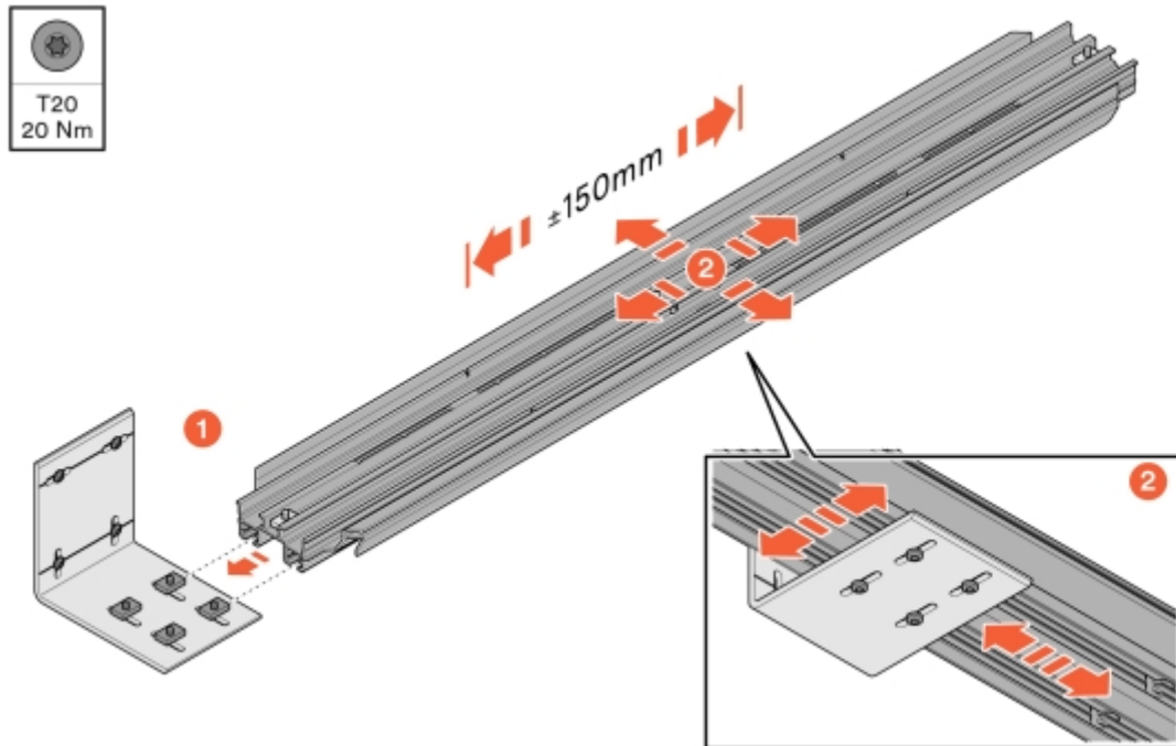
Illustration 31: Montage d'un support
