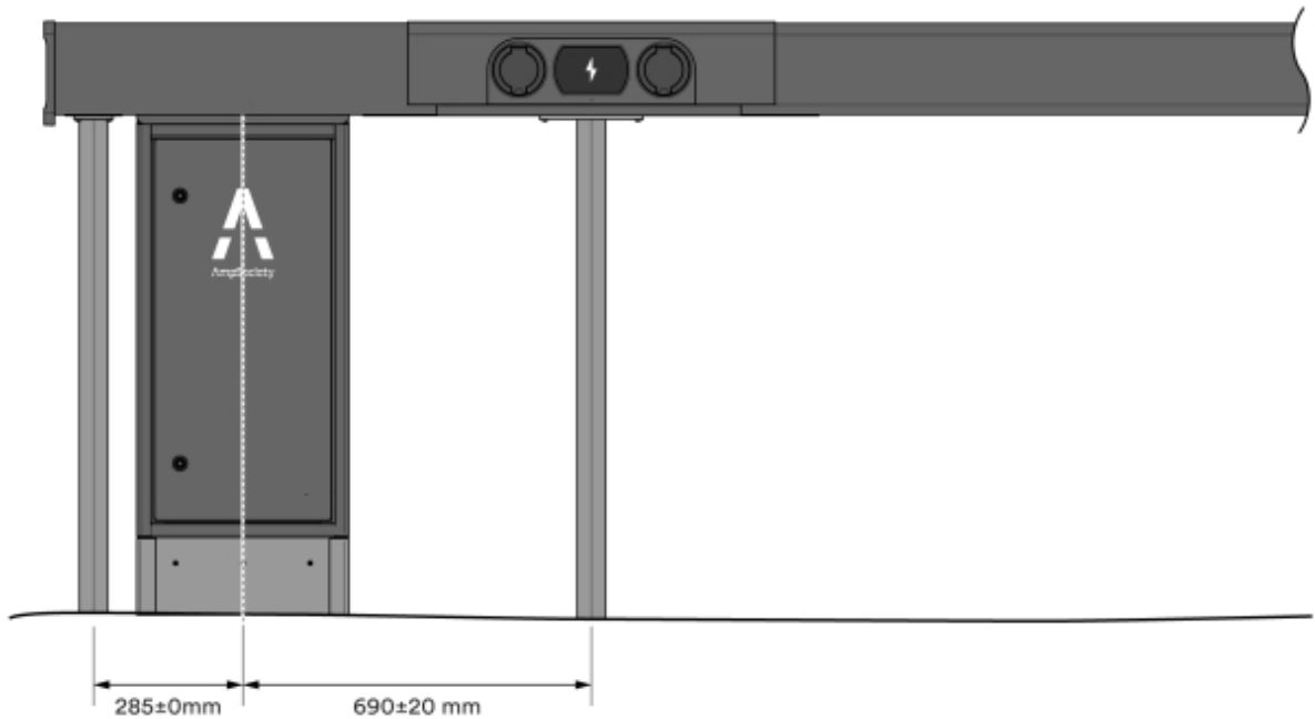
Illustration 7: Cotes - une seule direction
