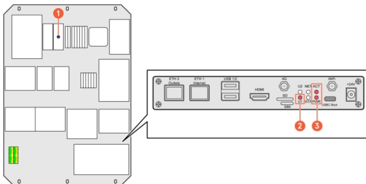
Illustration 43: Composants du SmartHub
