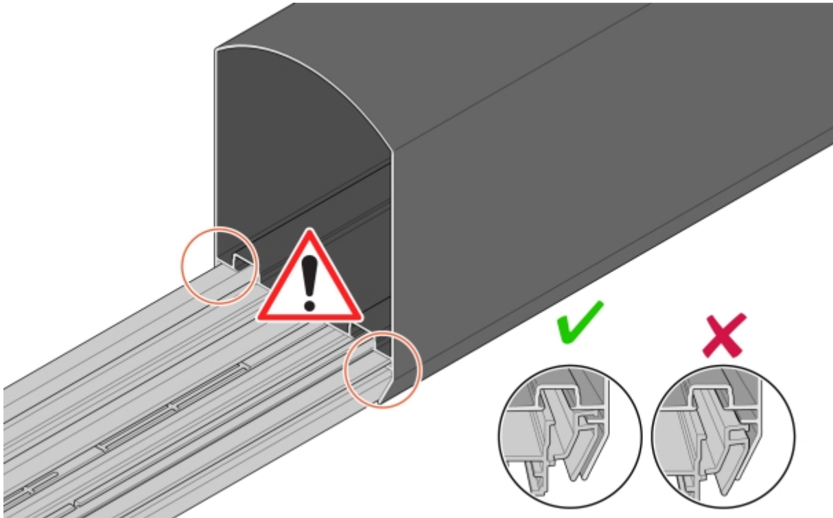
Illustration 21: Contrôle du montage
