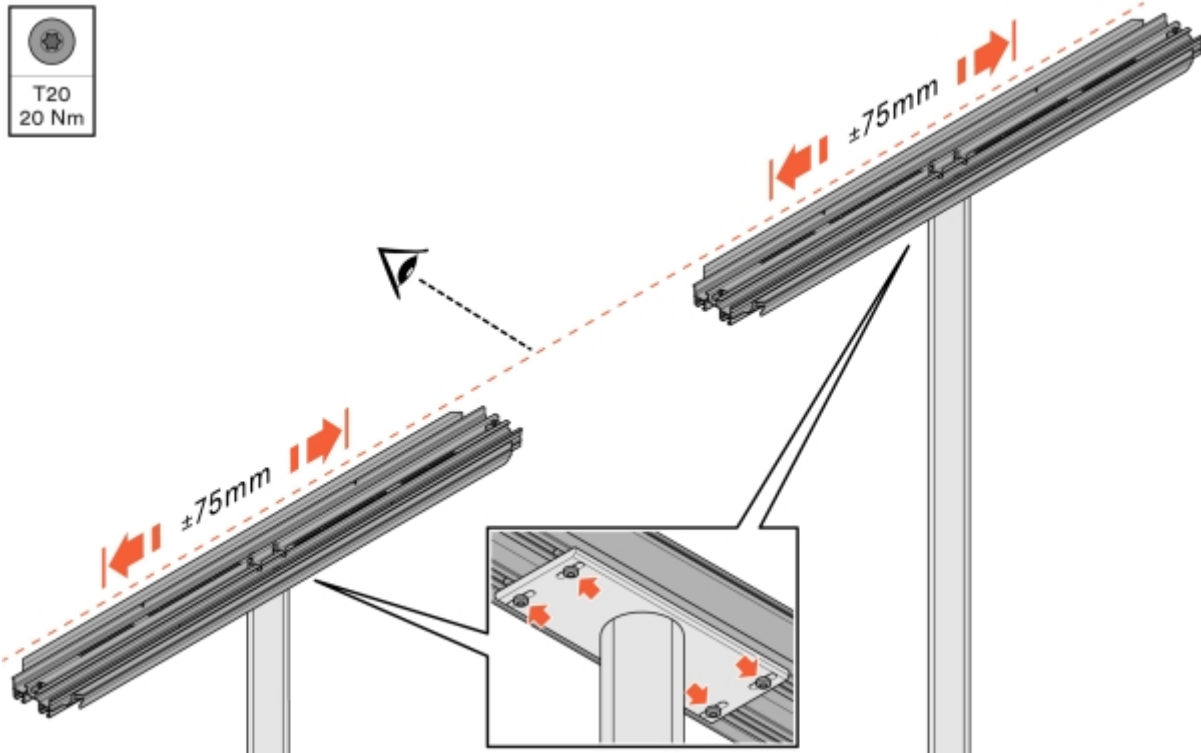
Illustration 19: Alignement et fixation d'un support
