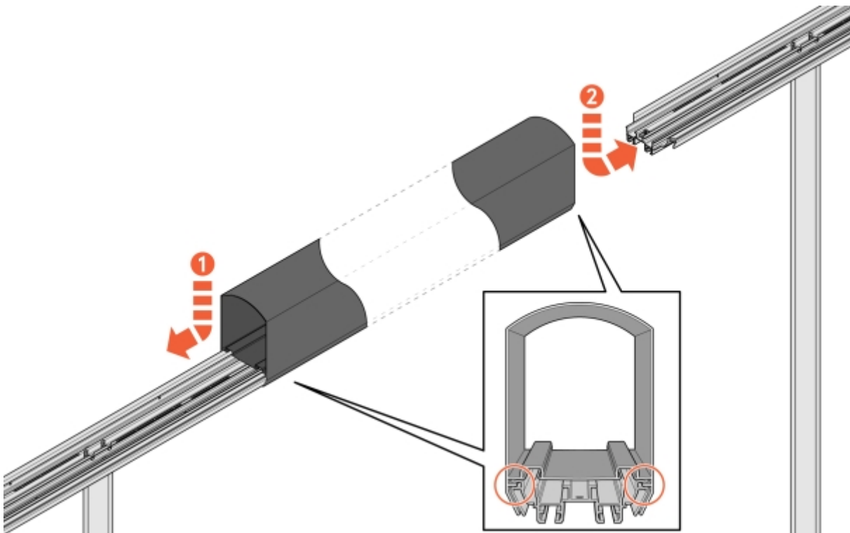
Illustration 20: Montage de la ConnectBar
