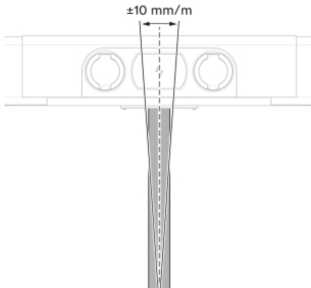
Illustration 15: Inclinaison maximale – latérale
