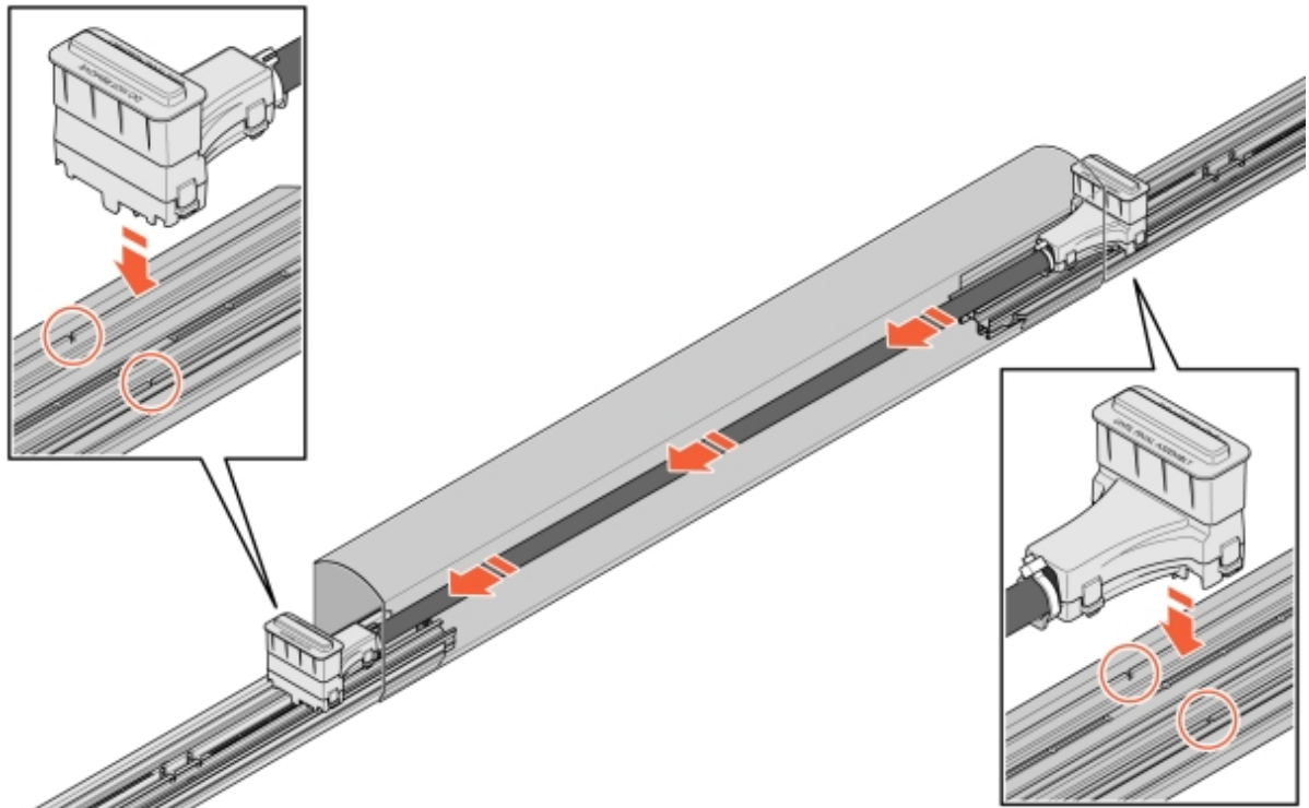
Illustration 39: Câblage dans la ConnectBar
