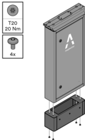
Illustration 6: Montage de la jupe de recouvrement
