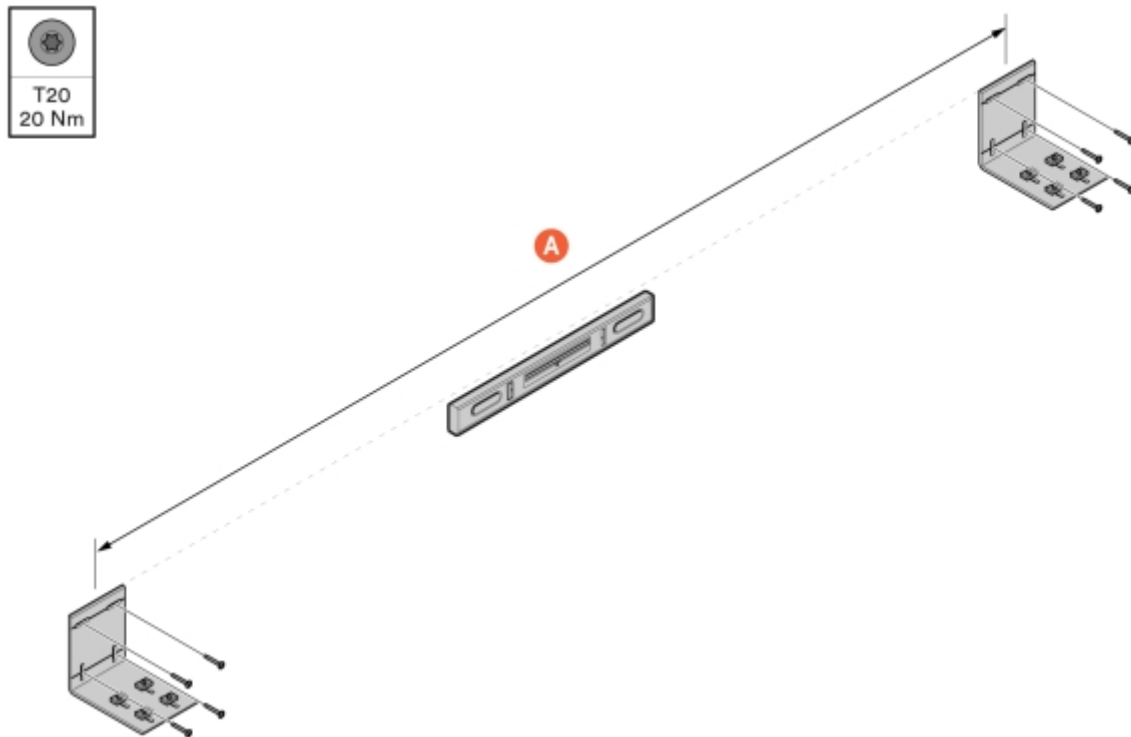
Illustration 30: Montage des fixations murales
