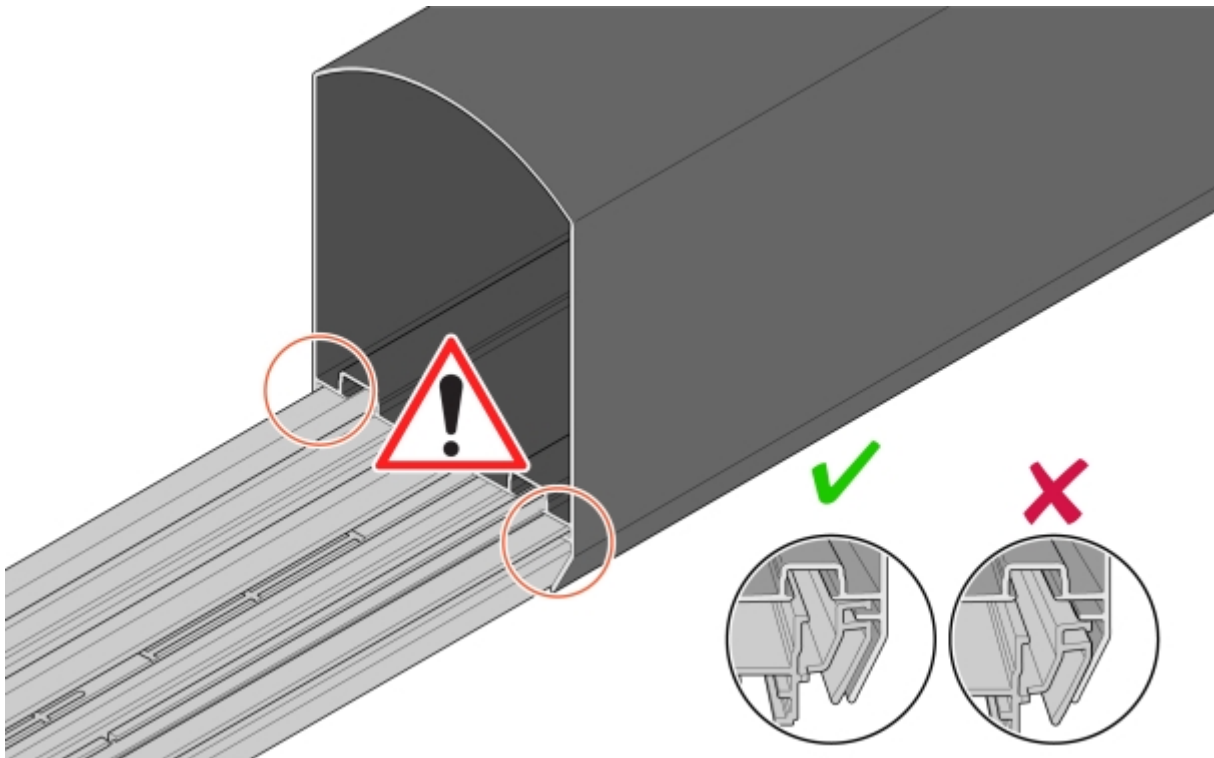
Illustration 34: Contrôle du montage
