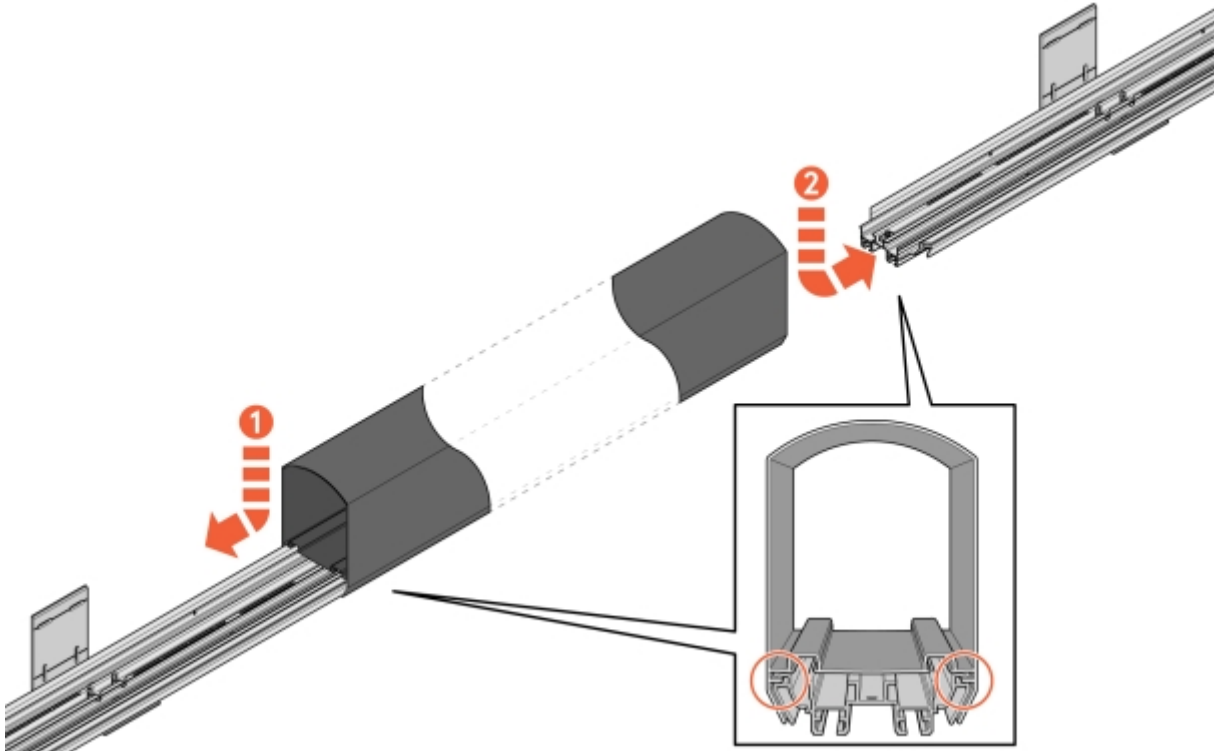
Illustration 33: Montage de la ConnectBar
