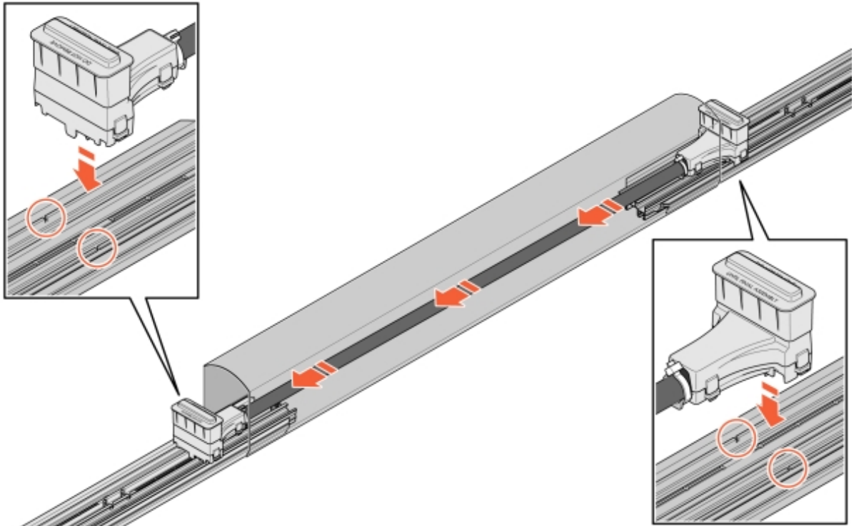
Illustration 26: Câblage dans la ConnectBar
