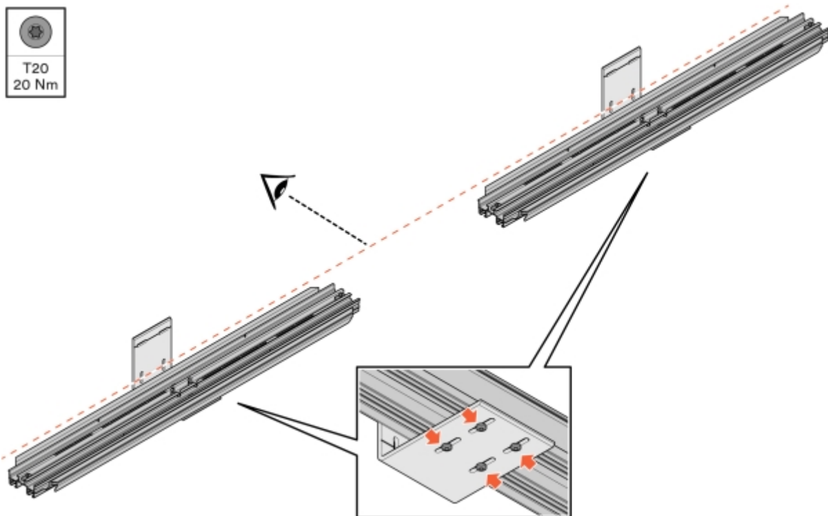
Illustration 32: Alignement et fixation d'un support
